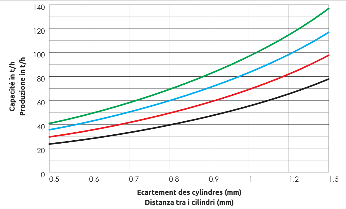
Capacité en t/h en fonction de l'écartement des cylindres Capacità in t/h in funzione della distanza tra i cilindri
