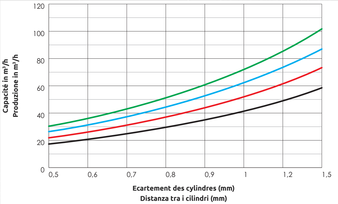
Capacité en [m³/Std.] en fonction de l'écartement des cylindres Capacità in m³/h secondo la distanza tra i cilindri
